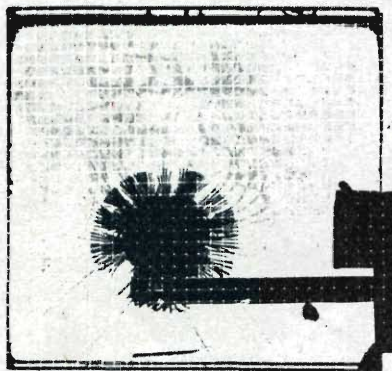
Sotto: Effetti di deflagrazione ottenuti da una macchina a ripresa rapida: nella loro progressione drammatica i fotogrammi mostrano chiaramente lo svilupparsi della forza esplosiva. Sopra: Foto di un modello di aereo bi-statoreattore, ripreso con il sistema ultrarapido, metodo delle ombre, senza banco ottico: in questo caso la velocità ultrasonica si è fatta statica.
