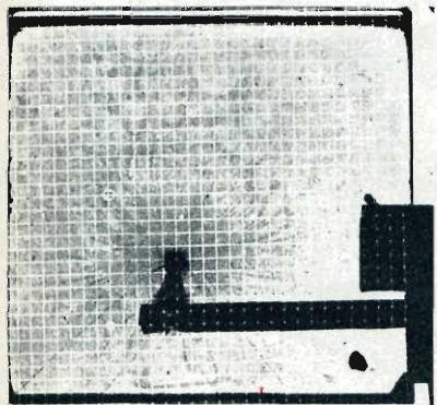
Sotto: Effetti di deflagrazione ottenuti da una macchina a ripresa rapida: nella loro progressione drammatica i fotogrammi mostrano chiaramente lo svilupparsi della forza esplosiva. Sopra: Foto di un modello di aereo bi-statoreattore, ripreso con il sistema ultrarapido, metodo delle ombre, senza banco ottico: in questo caso la velocità ultrasonica si è fatta statica.
