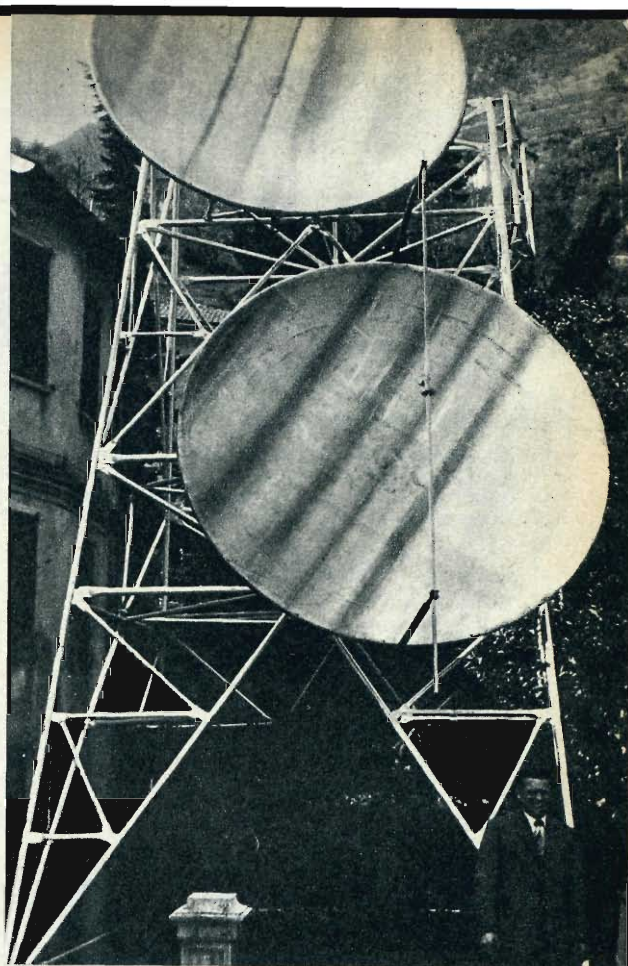
Torre di supporto delle antenne paraboliche: quelle illustrate nella foto sono sistemate sul Monte Colmenacco per il collegamento del tratto Como-Arsego. L'antenna inferiore ha già montato l'illuminatore con il ferro di guidaonda.
