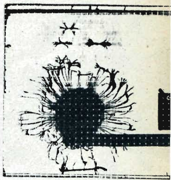
Sotto: Effetti di deflagrazione ottenuti da una macchina a ripresa rapida: nella loro progressione drammatica i fotogrammi mostrano chiaramente lo svilupparsi della forza esplosiva. Sopra: Foto di un modello di aereo bi-statoreattore, ripreso con il sistema ultrarapido, metodo delle ombre, senza banco ottico: in questo caso la velocità ultrasonica si è fatta statica.
