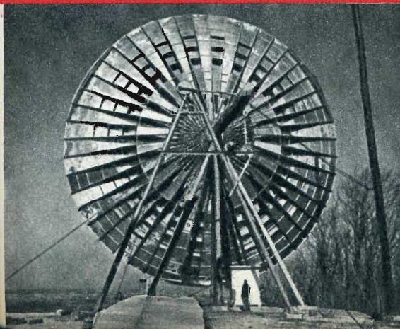
La fase di orientamento zenitale ed azimutale. A destra: L'antenna discoidale di circa 18 metri di diametro che la TV americana ha installato in Florida per il collegamento con l'isola di Cuba che fino ad oggi è priva di televisione.
